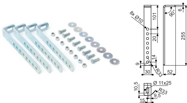
Vertikálne oceľové konzoly pre plastové skrinky Vertical steel brackets for plastic toolboxes
