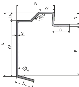
Obvodový oceľový profil Frame steel profile
