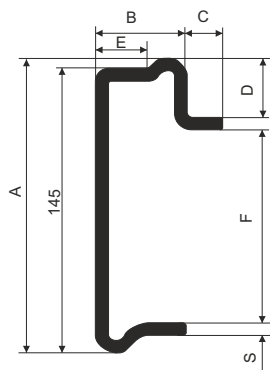
Obvodový oceľový profil Frame steel profile
