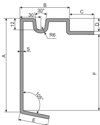
Obvodový oceľový profil Frame steel profile
