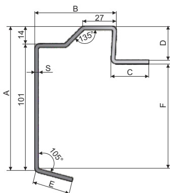
Obvodový oceľový profil Frame steel profile
