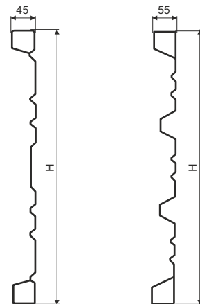
Bočnice hrúbka 1,5 - 2 mm
