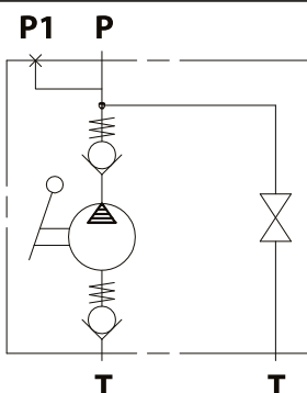
Hydraulická schéma Hydraulic layout
