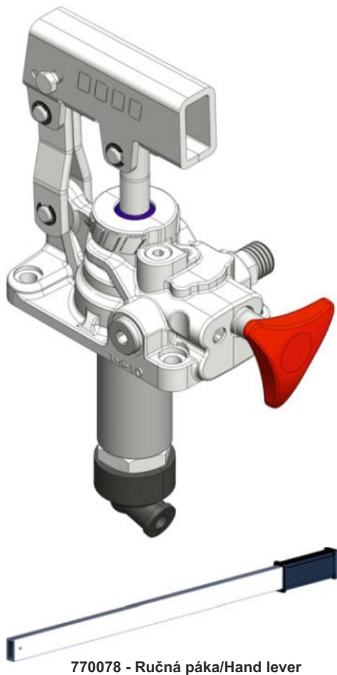
770078 - Ručná páka/Hand lever
