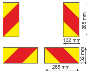
Obr. 2: Sada 4 reflexných tabúľ pre nákladné vozidlo Kit 4 truck panels
