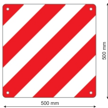
Kód 990032 Hliníkové tabule 500x500x1mm s červeným pruhovaním triedy 1 a matnou bielou farbou Aluminium panel 500x500x1mm red film class 1 and white mat ink.
