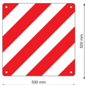
Kód 990034 Hliníkové tabule 500x500x1mm červeno-bielo pruhované s 4 dierami a zaokrúhlenými okrajmi Aluminium panel 500x500x1 mm film class 1 with four riveted holes and rounded corner
